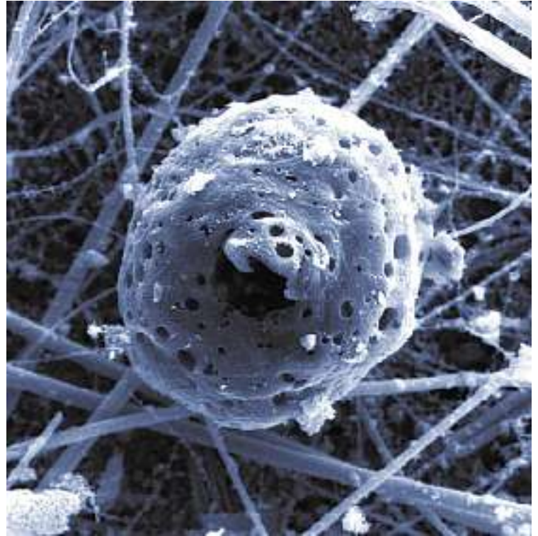
Dieselmrußpartikel, stark vergrößert.
